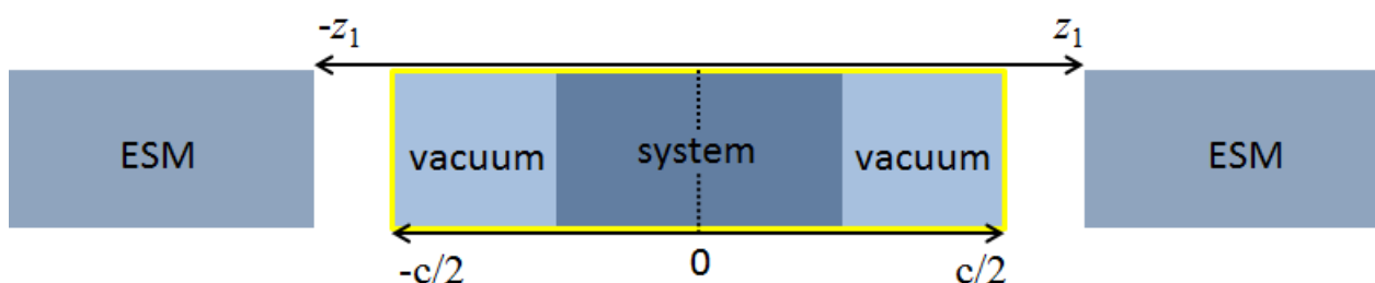
図 5.3-7 ESM 法において仮定している原子配置の定義方法の模式図
