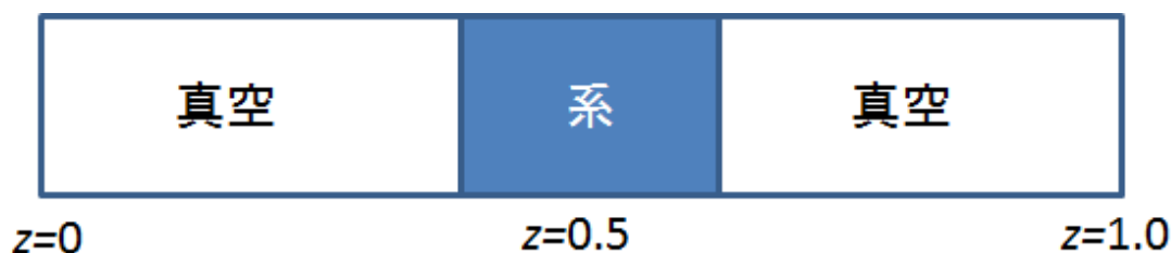
図 5.3-10 Dipole 補正を有効にする表面系の模式図
