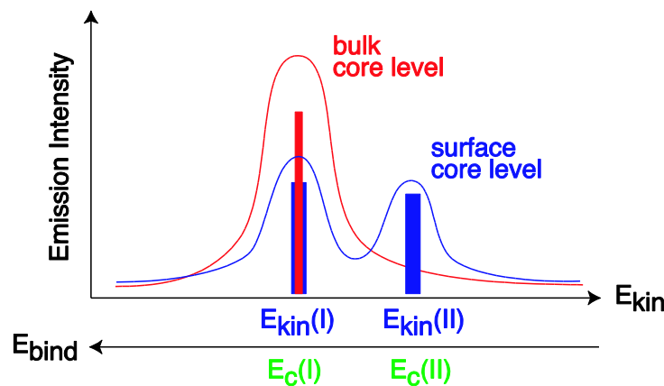
図 5.1-12 内殻光電子放出のスペクトル
