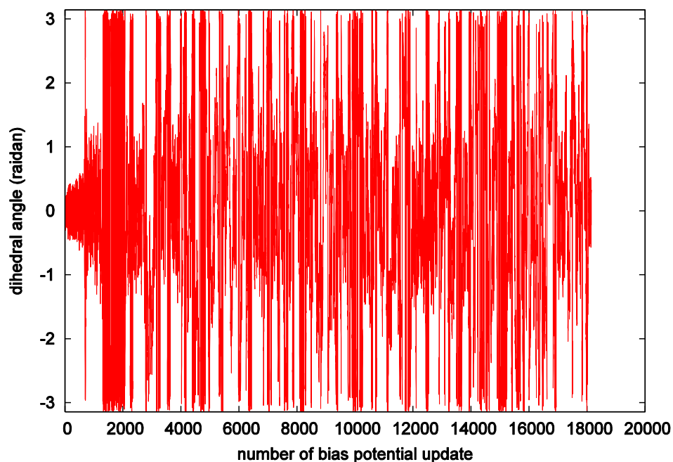
図 5.4-12 2 面角とバイアスポテンシャル更新回数との関係
