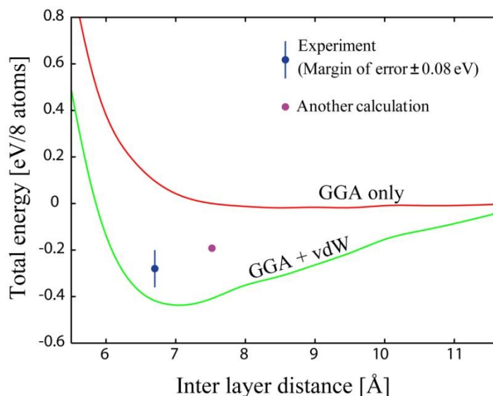
図 5.3-6 積層グラファイトの全エネルギーの層間距離依存性. GGA (赤線) と GGA+vdW (緑線) による比較
