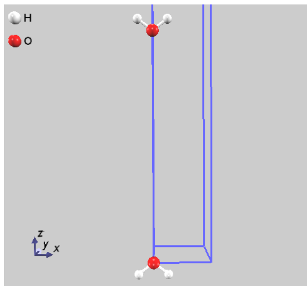
図 5.3-8 H 2 O 分子を互い違いに配置した系。
