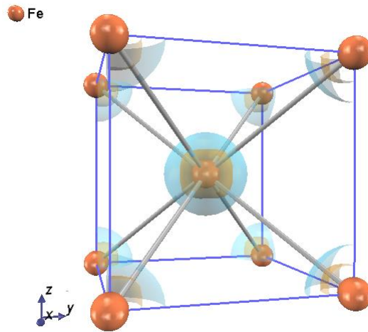
図 4.11 Fe の電荷密度分布図. 青色とオレンジ色の面は, 自発磁化により生じた, 多数派スピンの多数派スピンと少数派スピンの少数派スピンによる 電荷密度分布の等値面を表す.
