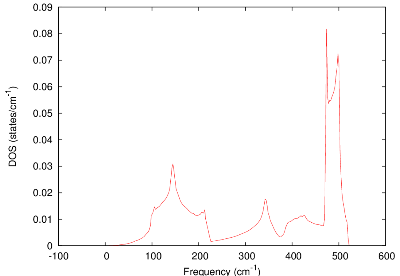
図 5.2-8 シリコン結晶のフォノン状態密度。
