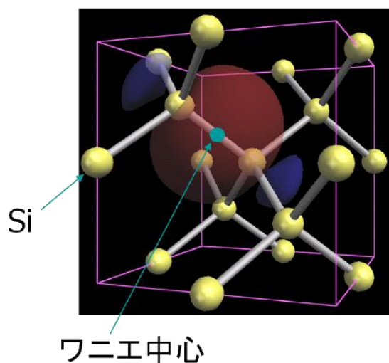
図 5.1-7 Si 結晶(a)と GaAs 結晶(b)の最大局在ワニエ関数
