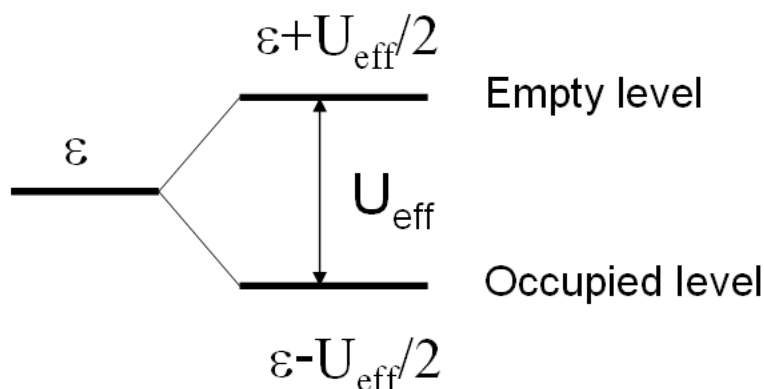
図 5.3-1 ハバード補正による軌道エネルギーの変化
