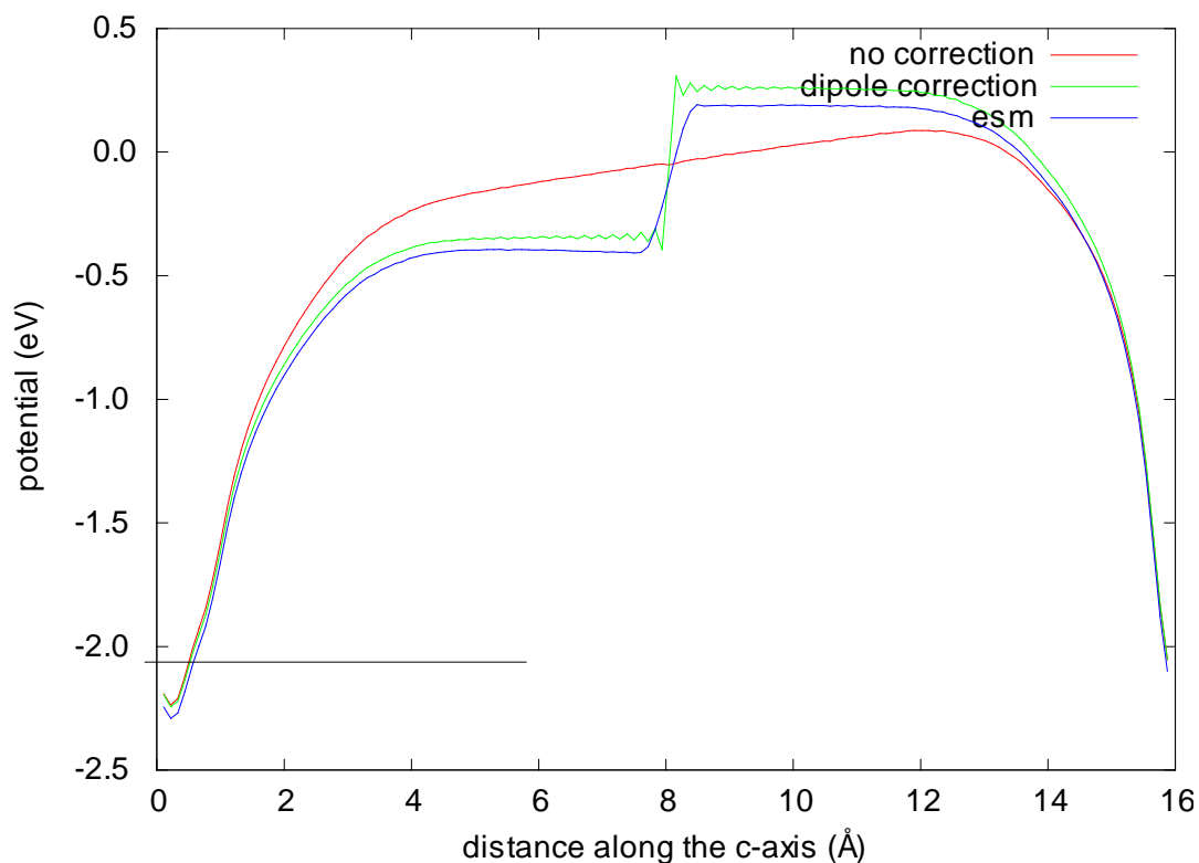
図 5.3-11 真空層と局所ポテンシャルの関係
