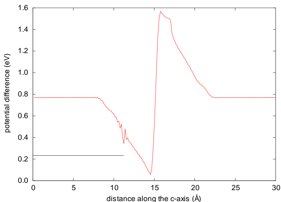
図 5.3-9 ローカルポテンシャルの差分と表面に垂直な距離との関係。
