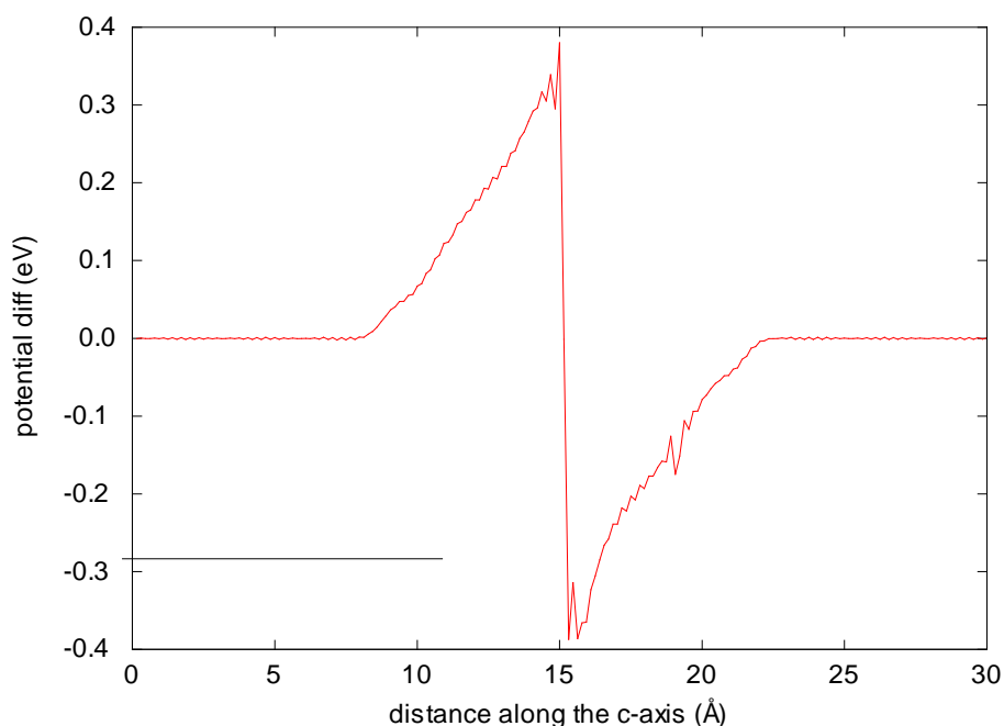
図 5.3-12 ローカルポテンシャルの差分と表面に垂直な距離との関係。
