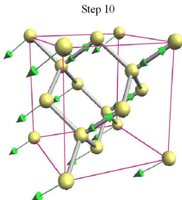
図 9.7-2 ブラベーセルで表したバルク Si の構造最適化過程(step 10)
