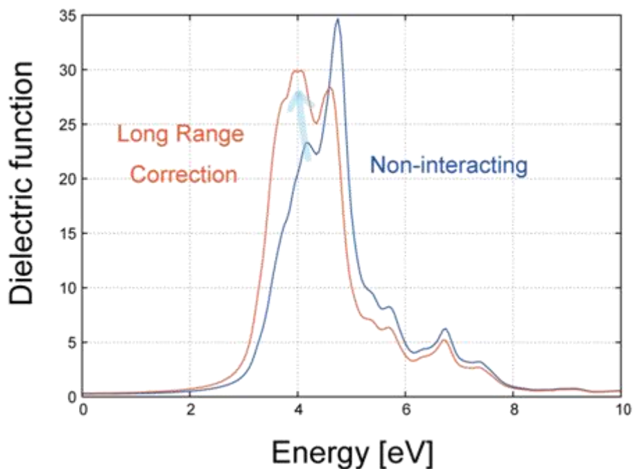
図 11.6-1 LRC による Si 結晶誘電スペクトルの変化。青線は独立粒子近似による結果。
