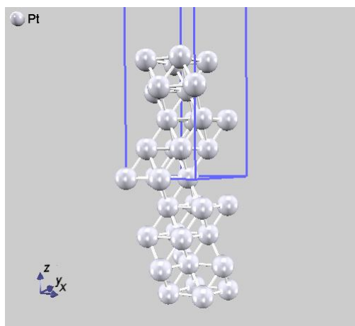
図 4.5-2 Pt(111) 面の原子配置。表面モデルの中央を原点にすることによって反転対称性がある。
