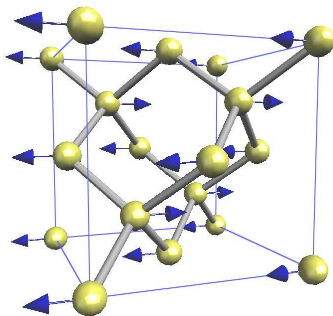
図 9.9-1 バルク Si の基準振動の固有ベクトル
