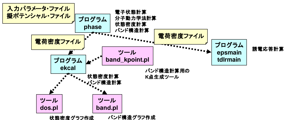
図 1.2-1 PHASE/0 のプログラム構成
