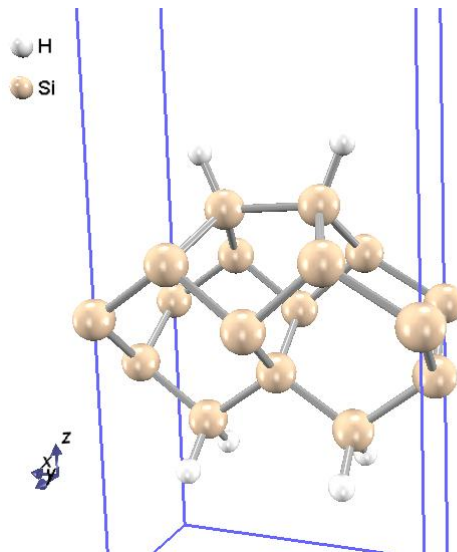
図 4.5-1 水素終端した Si(001)-p(2×1) 表面の構造図
