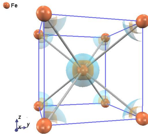
図 4.7-1 Fe の電荷密度分布図. 青色とオレンジ色の面は, 自発磁化により生じた, 多数派スピンの多数派スピンと少数派スピンの電荷密度分布の等値面を表す.
