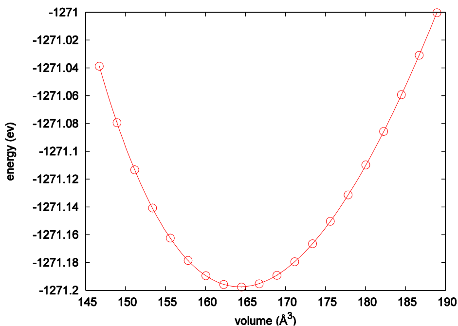
図 4.10-1 シリコンの Energy-Volume 曲線。白丸は計算値、実線はフィットした結果。
