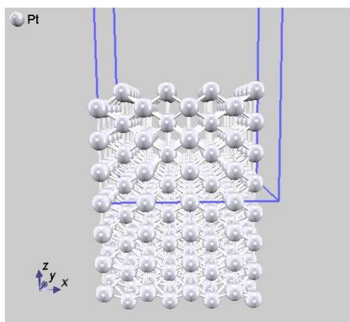
図 4.5-3 Pt(110) 理想表面(スーパーセル表示)
