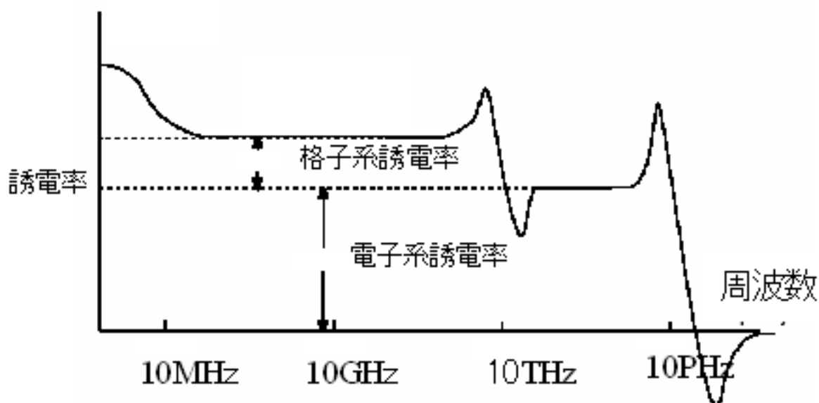
図 11.1-1 誘電率の誘電分散
