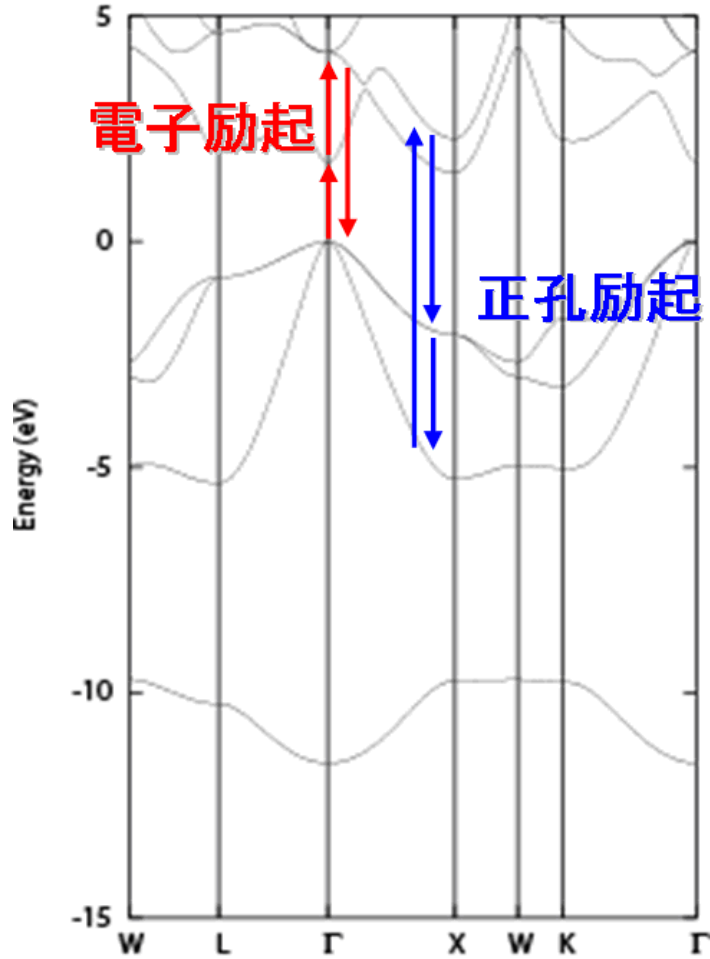
図 11.2-1 SHG 過程における電子と正孔の仮想励起
