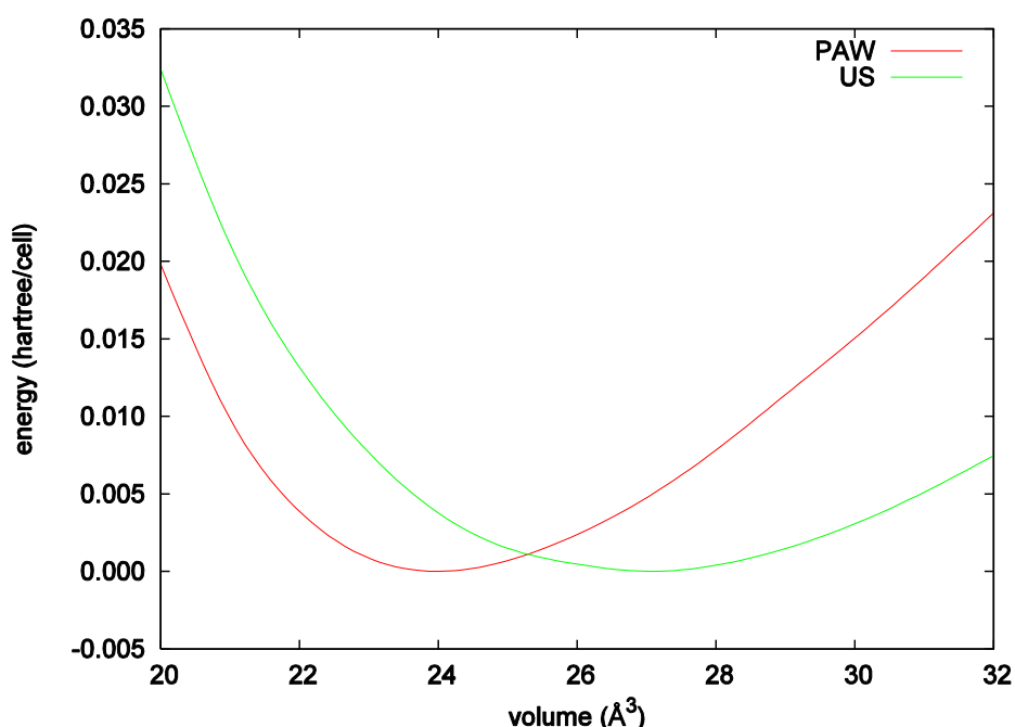
図 6.3-1 クロムの EV 曲線。赤線が PAW の結果、緑線が US の結果。各手法で得られた最も低いエネルギーをエネルギーの原点としている。
