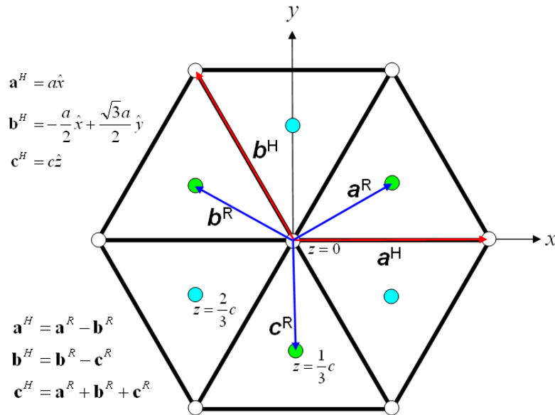
図 4.2-1 六方晶系と菱面体晶系の関係. 六方軸の方から見た格子点と基本並進ベクトルが示されています.
