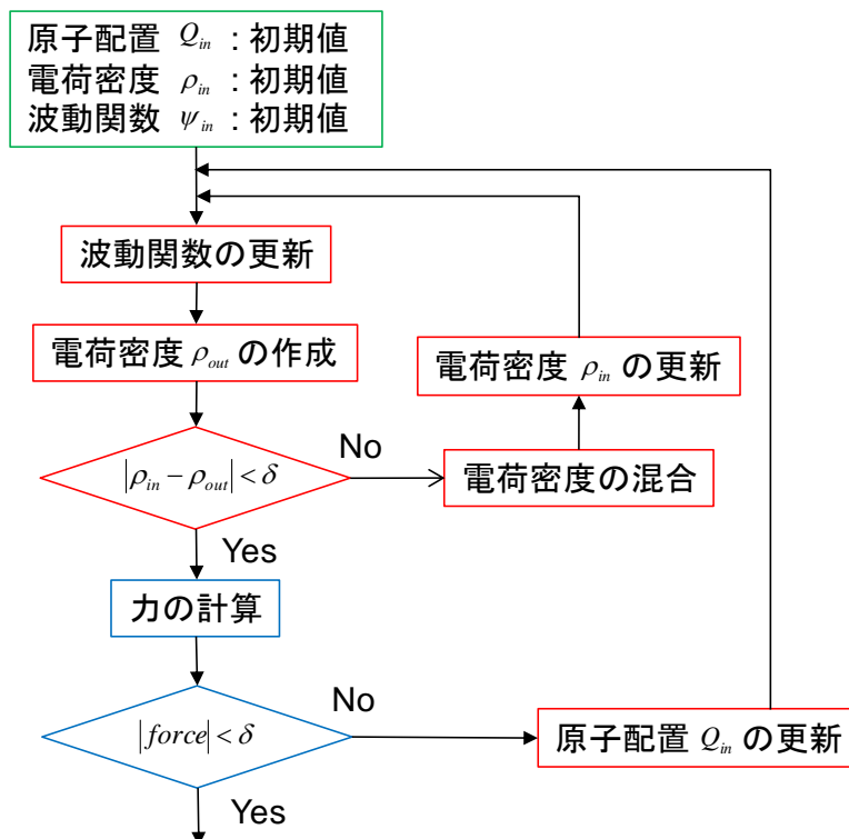
図 3.6-1 PHASE における計算フロー
