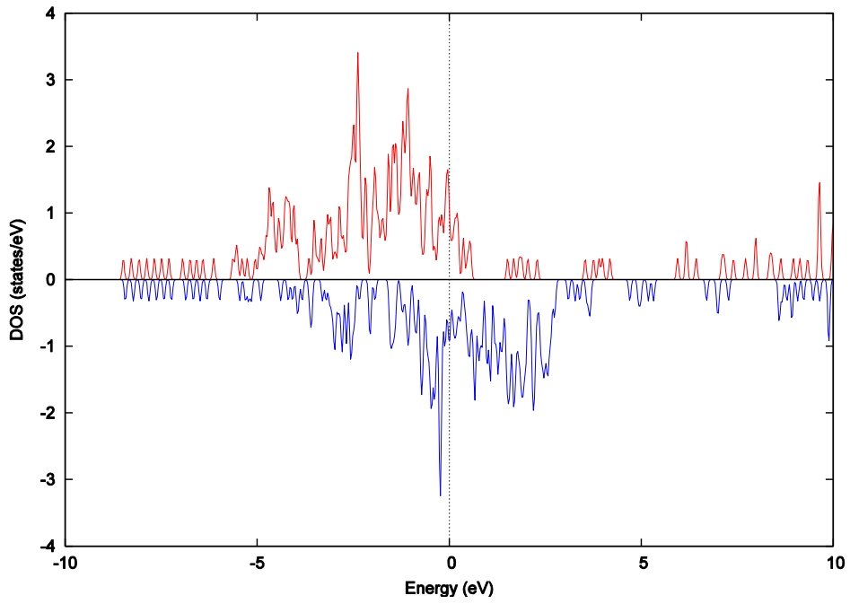
図 4.8-1 Gaussian 法で計算した体心立方鉄の状態密度
