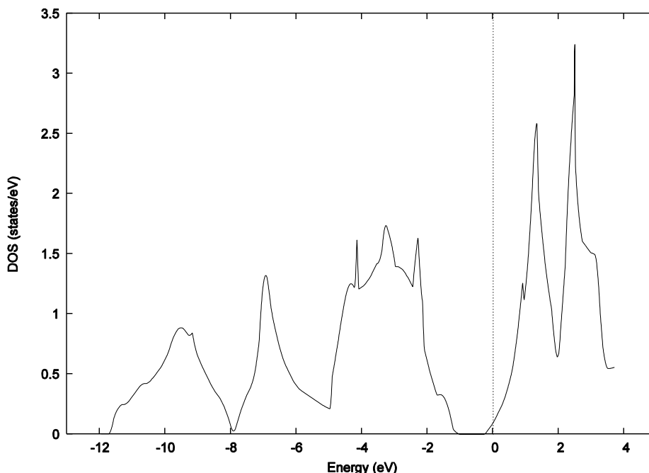
図 4.2-3 Si 2 の状態密度
