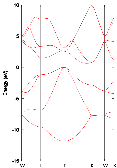
図 2.5-2 バンド構造 可視化例 (Si ダイヤモンド構造のバンド構造)
