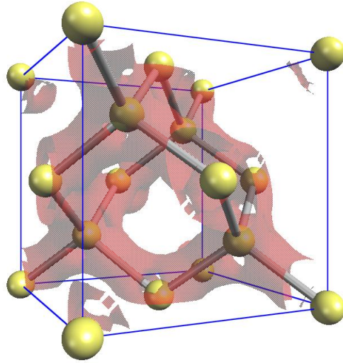
図 4.1-2 シリコン結晶の電荷密度分布
