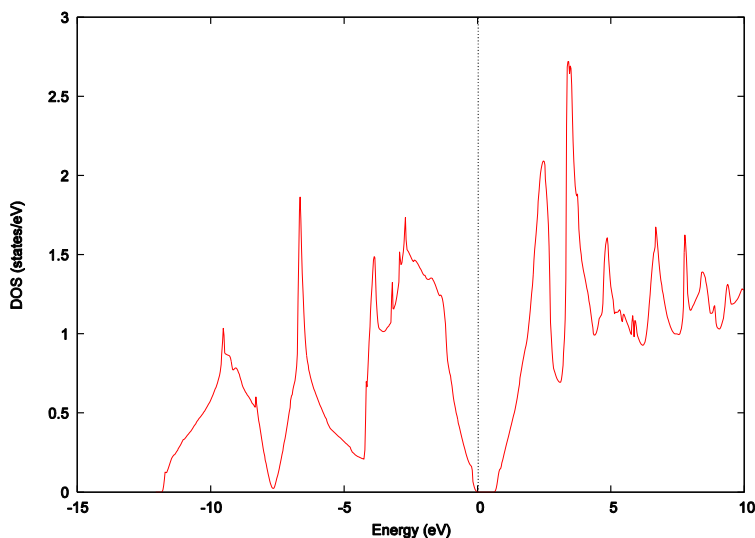
図 2.5-1 状態密度 可視化例 (Si ダイヤモンド構造のバンド構造)
