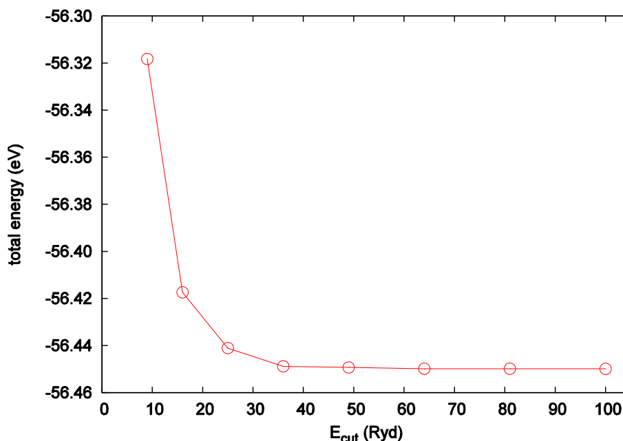
図 7.1-1 アルミニウム結晶の場合の、カットオフエネルギーと全エネルギーの関係
