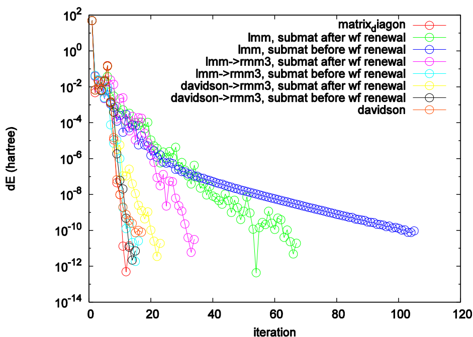
図 7.1-4 波動関数ソルバーによる収束の速さの比較
