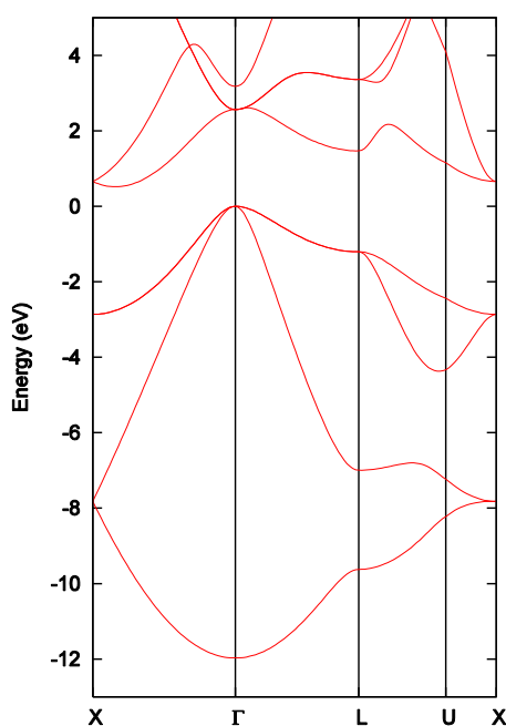
図 9.6-1 パルク Si のバンド構造図
