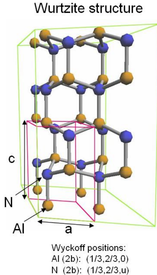
図 11.4-2 Wurtzite 構造の AlN
