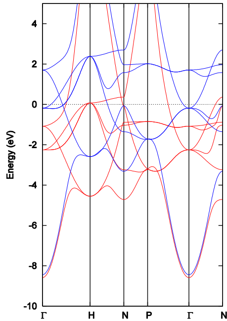
図 4.9-1 体心立方鉄のバンド構造図。
