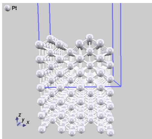
図 4.5-4 Pt(110) 面 missing-row 構造(スーパーセル表示)
