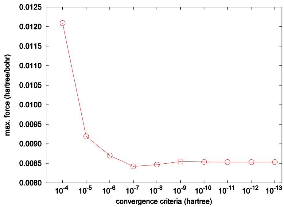
図 7.1-3 SiO 2 の、収束判定と力の最大値の関係
