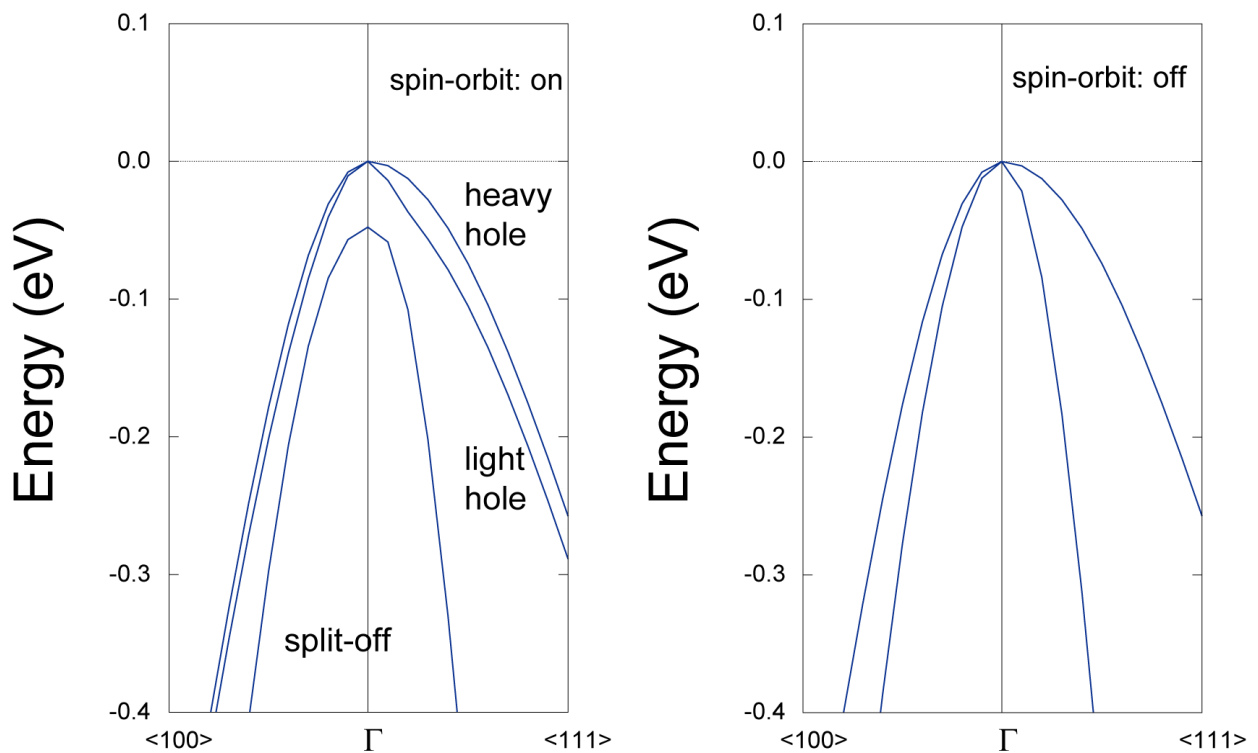
図 5.7-2 Si 結晶のバンド。(左)スピン軌道相互作用あり。(右)なし。
