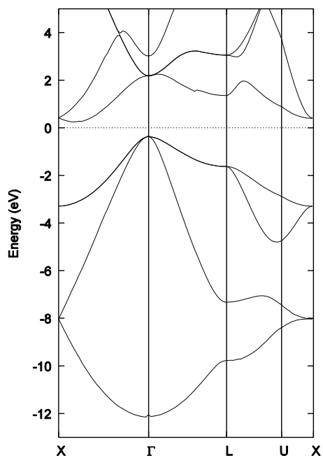
図 4.2-4 Si2 のバンド構造
