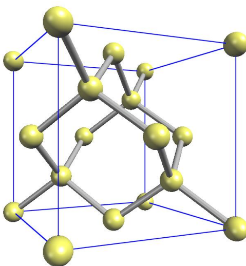
図 4.1-1 シリコン原子が構成するダイヤモンド構造
