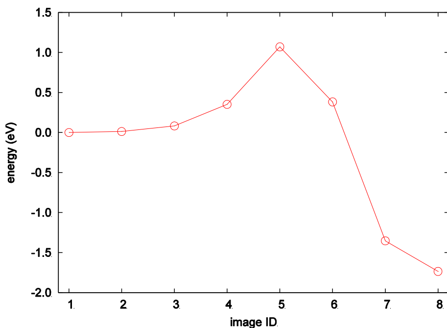
図 5.4-4 最終的に得られる反応経路と各レプリカのエネルギーの関係
