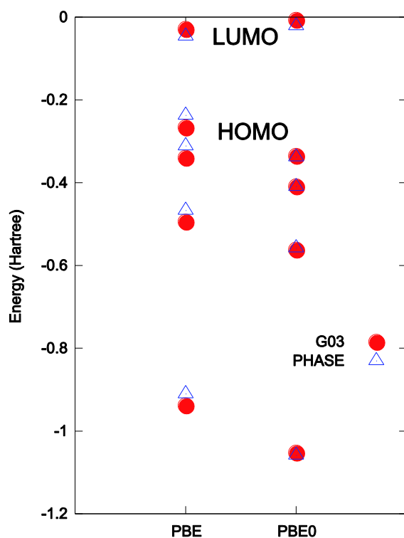
図 5.3-4 PBE 汎関数法, PBE0 汎関数法による水分子のエネルギー準位が Gaussian03 (G03) の結果と比較して示されている。
