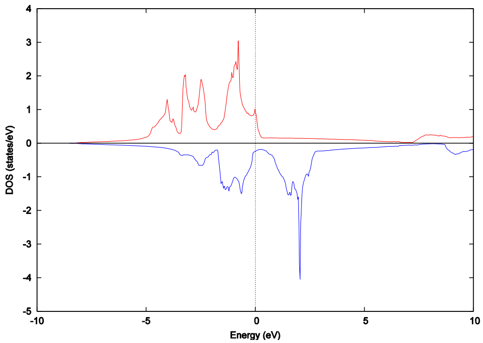
図 4.8-2 Tetrahedral 法で計算した体心立方鉄の状態密度
