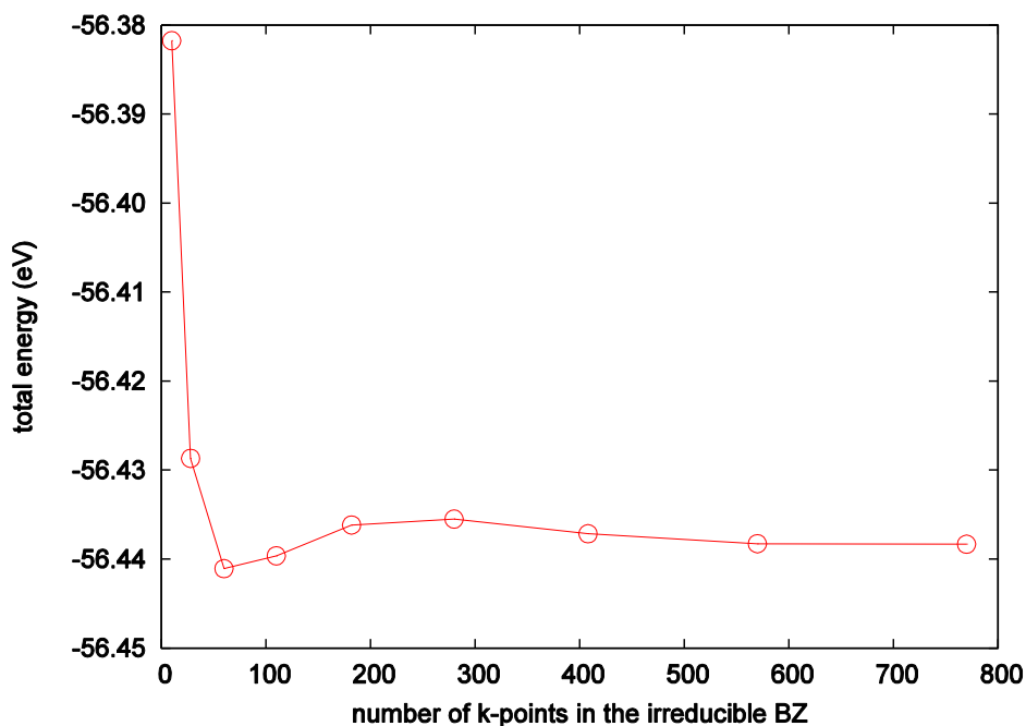
図 7.1-2 アルミニウム結晶の場合の、k 点数と全エネルギーの関係
