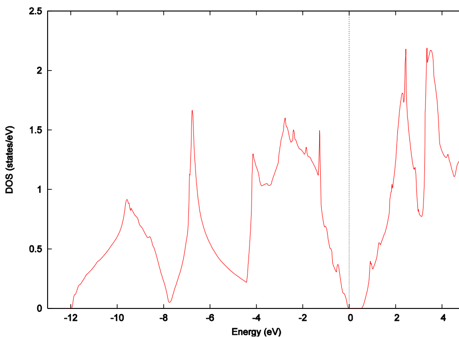
図 9.4-1 バルク Si の状態密度図
