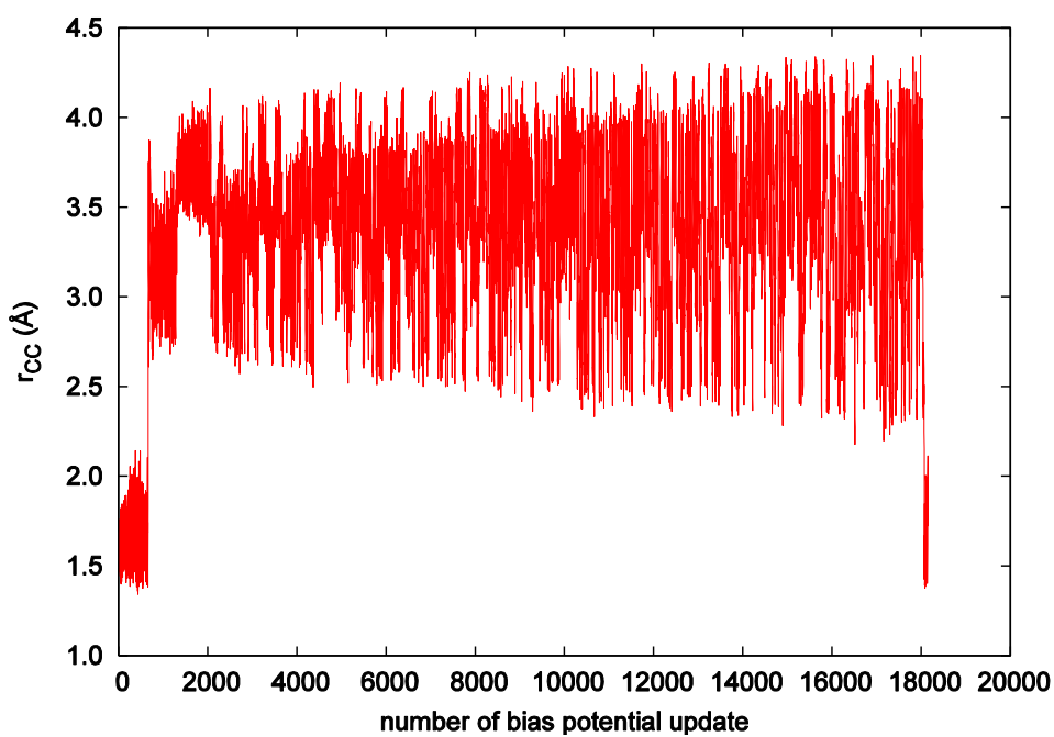
図 5.54 炭素原子間距離とバイアスポテンシャル更新回数関係
