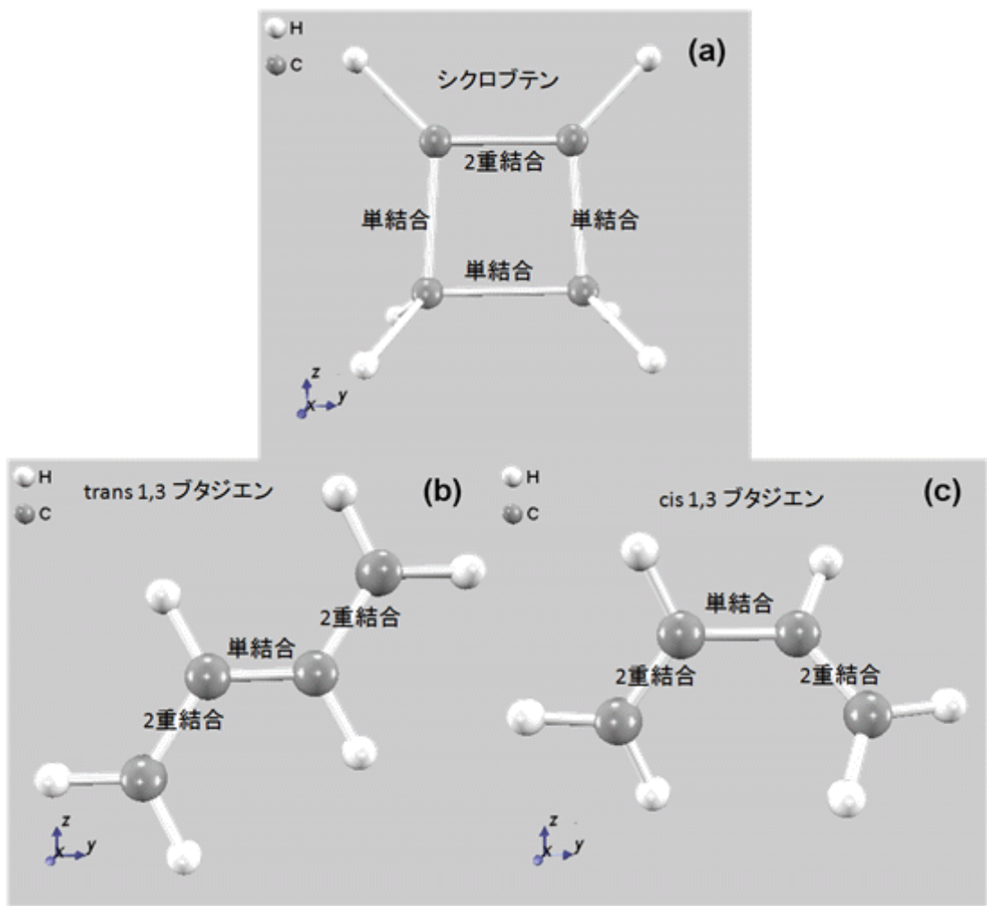
図 5.50 C_4H_6 分子の分子構造
