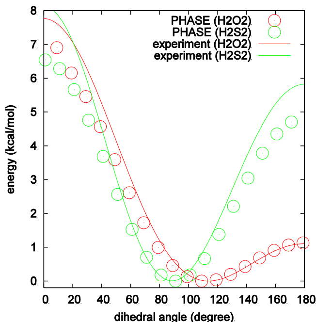
図 5.48 H 2 O 2 および H 2 S 2 分子の 2 面角とエネルギーの関係
