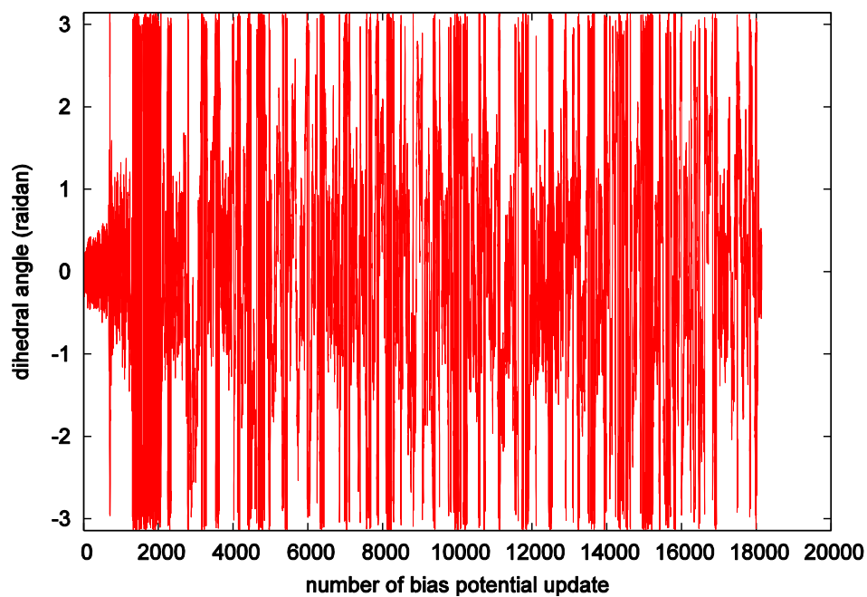
図 5.53 2 面角とバイアスポテンシャル更新回数の関係
