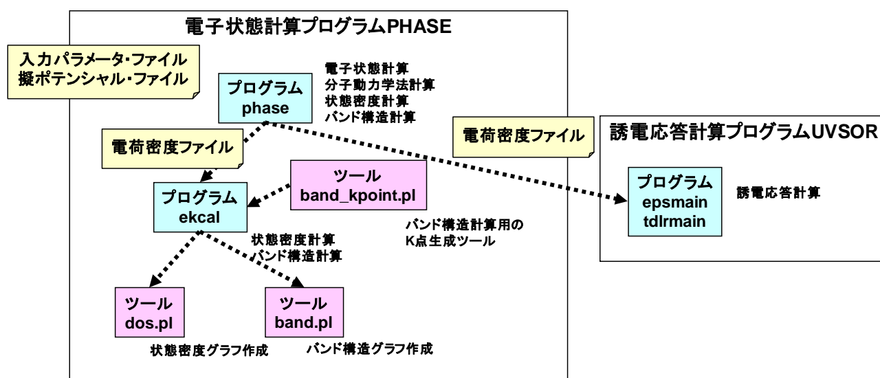
図 1.2 PHASE、UVSOR のプログラム構成
