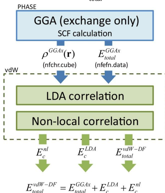
図 5.38 本ルーチン (vdW.F90) の計算の流れ
