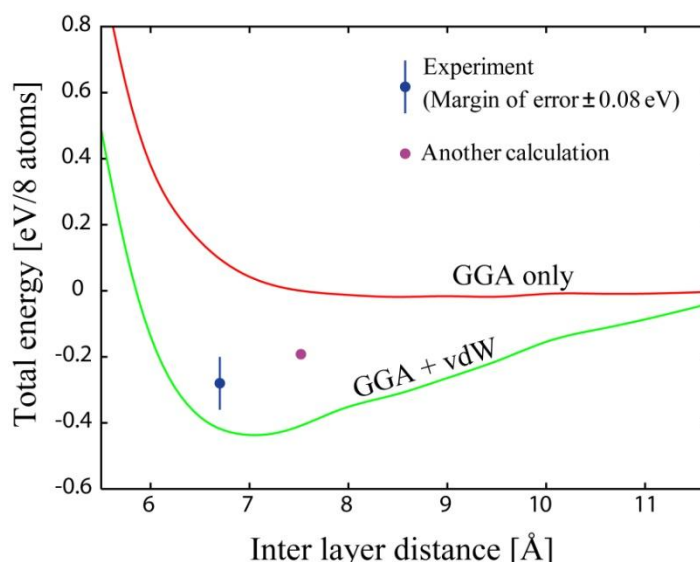
図 5.39 積層グラファイトの全エネルギーの層間距離依存性. GGA (赤線) と GGA + vdW (緑線) による比較
