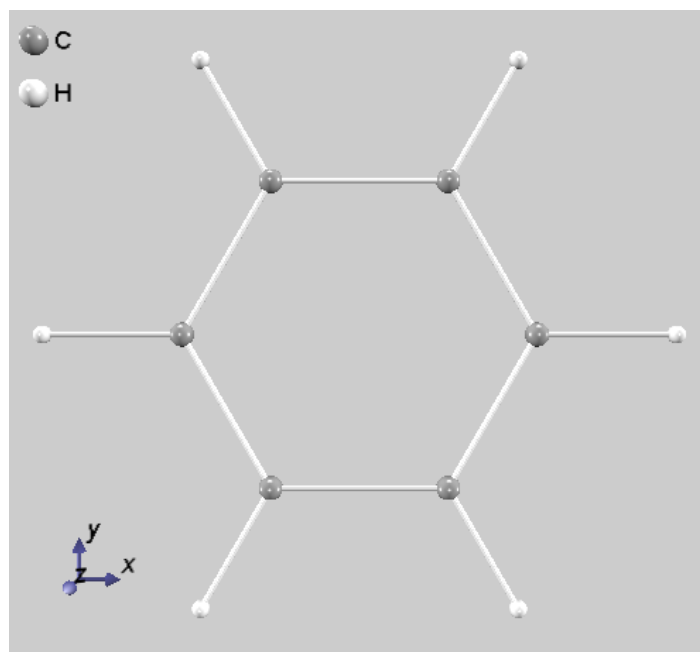
図 5.57 ベンゼン分子の原子配置
