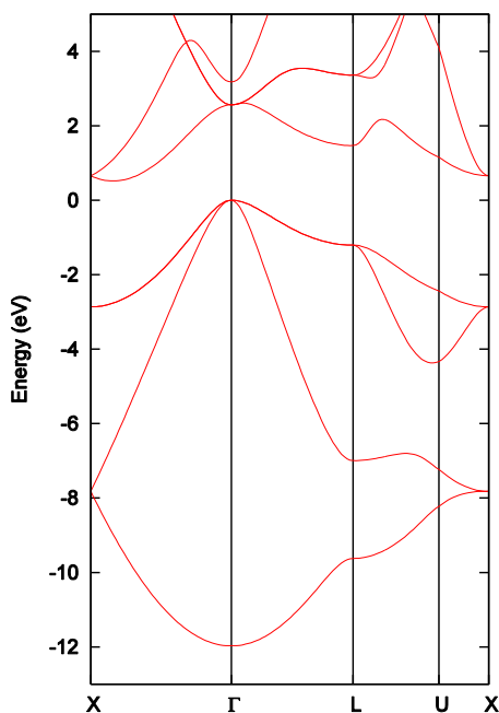
バルク Si のバンド構造図
