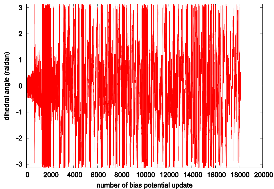
図 5.54 2 面角とバイアスポテンシャル更新回数の関係
