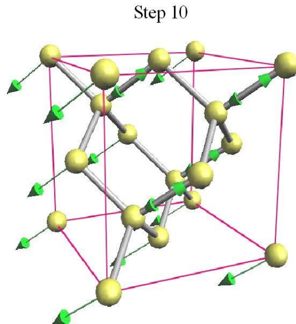
図 9.3 ブラベーセルで表したバルク Si の構造最適化過程(step 10)
