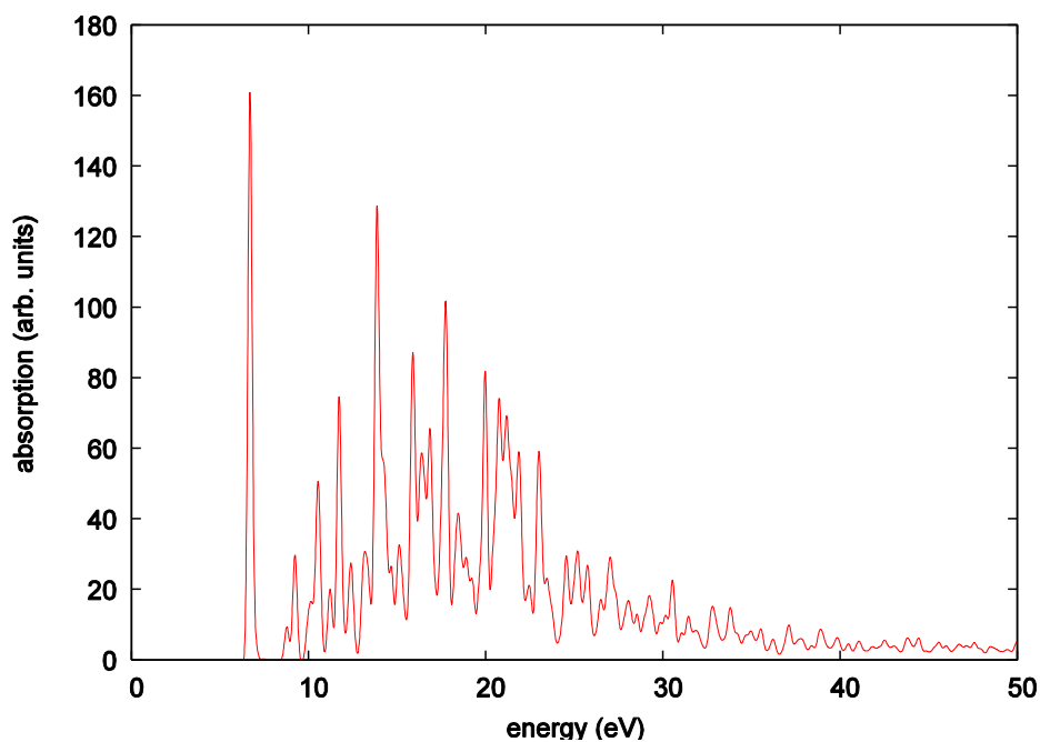
図 5.58 本例題によって得られる吸収スペクトル
