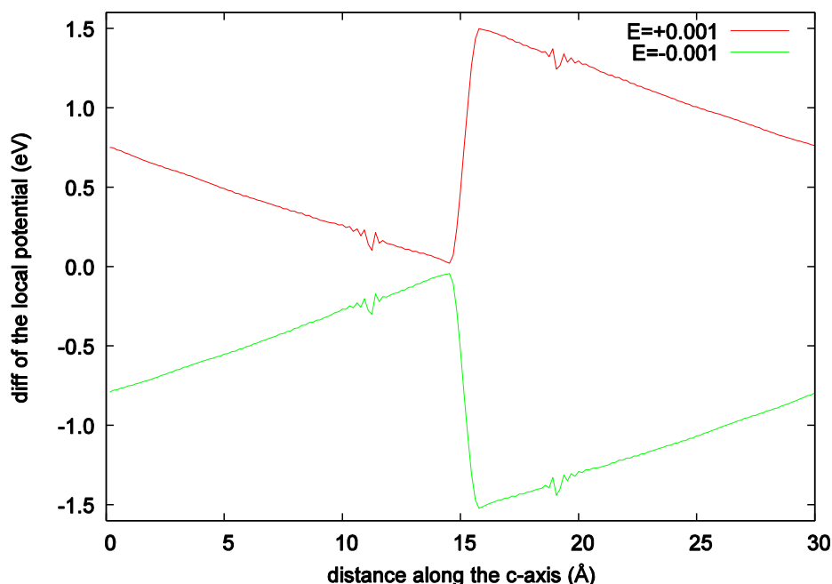
図 5.42 ローカルポテンシャルの差分と表面に垂直な距離との関係。赤線：電場が 0.001 のケース、緑線：電場が -0.001 のケース。
