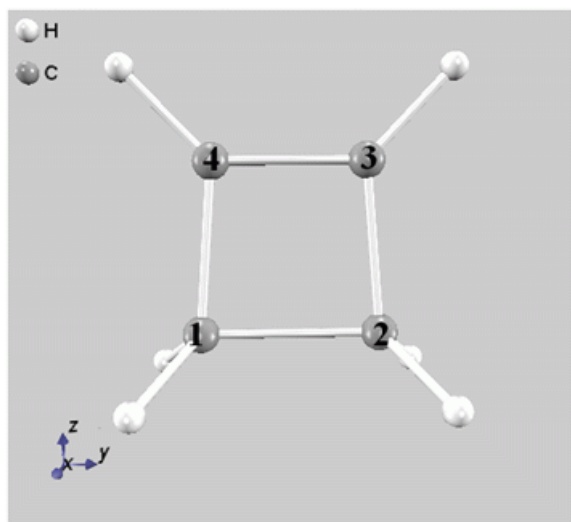
図 5.52 C_4H_6 分子の分子構造
