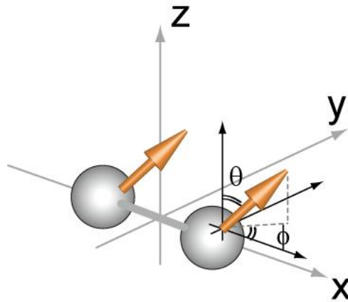
図 5.61 スピン軌道相互作用計算の計算例の分子配置
