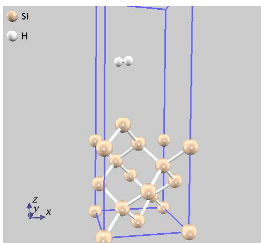
図 5.43 本例題の始状態
