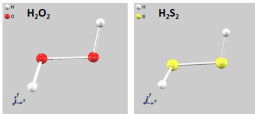
図 5.48 H 2 O 2 および H 2 S 2 分子の分子構造
