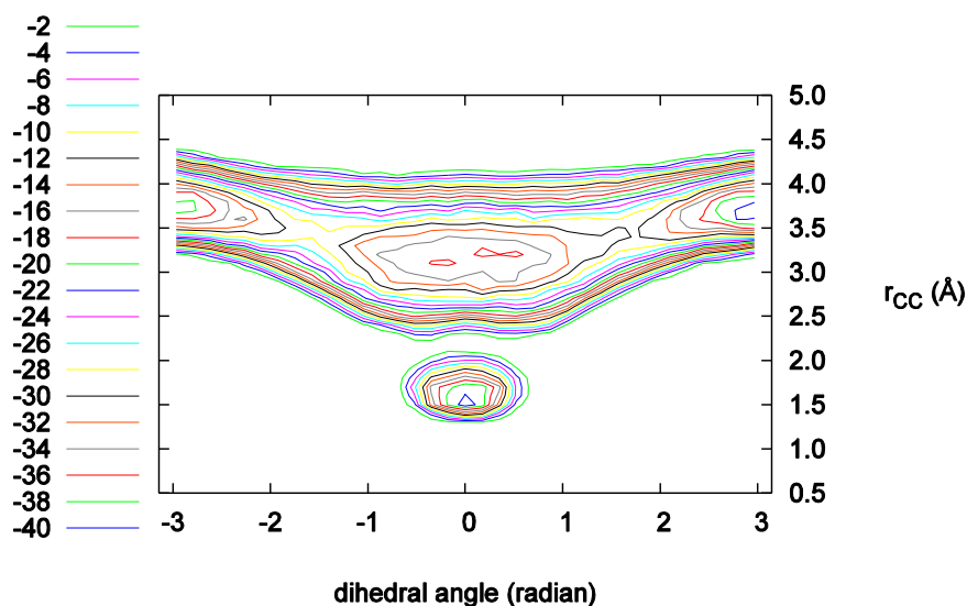
図 5.53 C 4 H 6 分子の自由エネルギー表面
