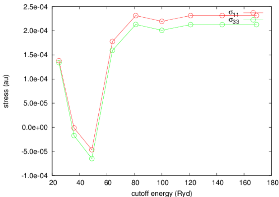
図 5.60 ルチル型 \text{TiO}_2 の場合の、ストレステンソルとカットオフエネルギーの関係
