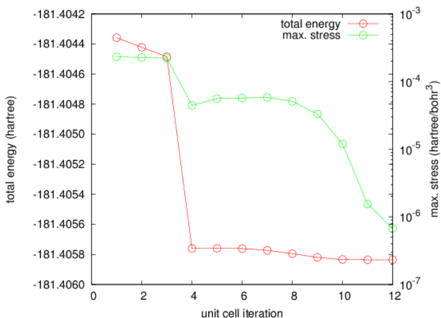
図 5.59 単位胞最適化の履歴。赤線：全エネルギー，緑線：ストレステンソルの最大成分。
