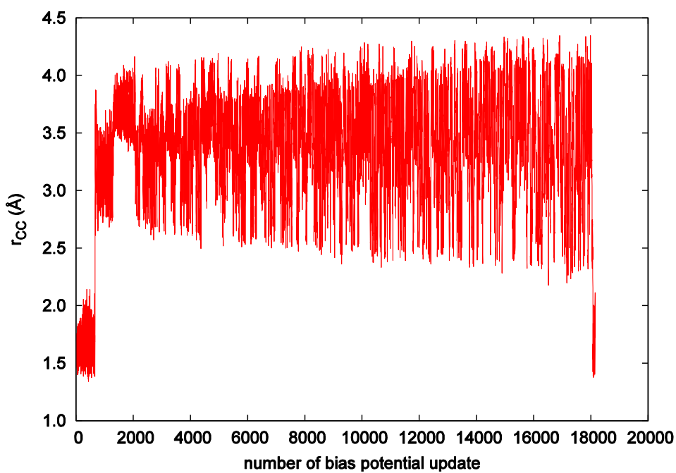
図 5.55 炭素原子間距離とバイアスポテンシャル更新回数関係
