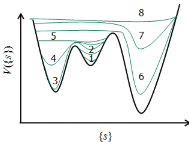
図 5.50 Meta-dynamics シミュレーションの様式図
