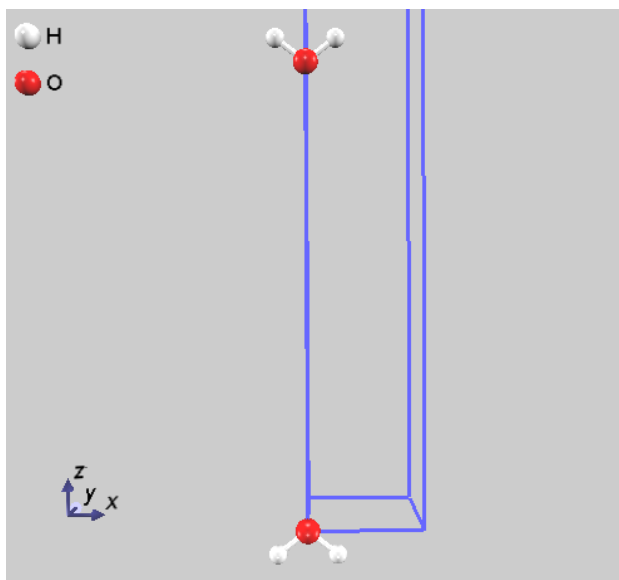
図 5.41 H 2 O 分子を互い違いに配置した系。
