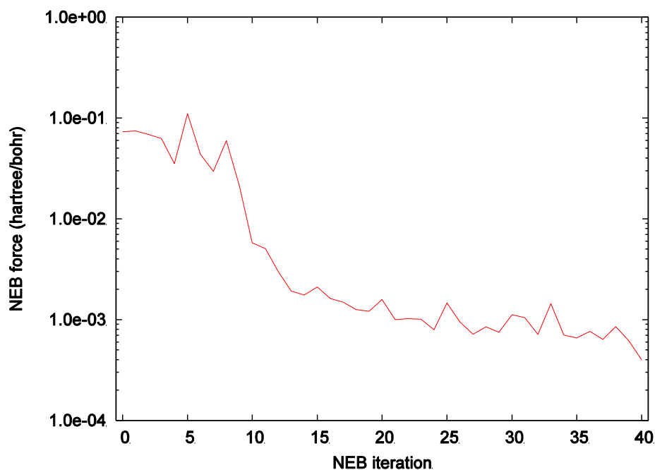
図 5.45 NEB 力の履歴
