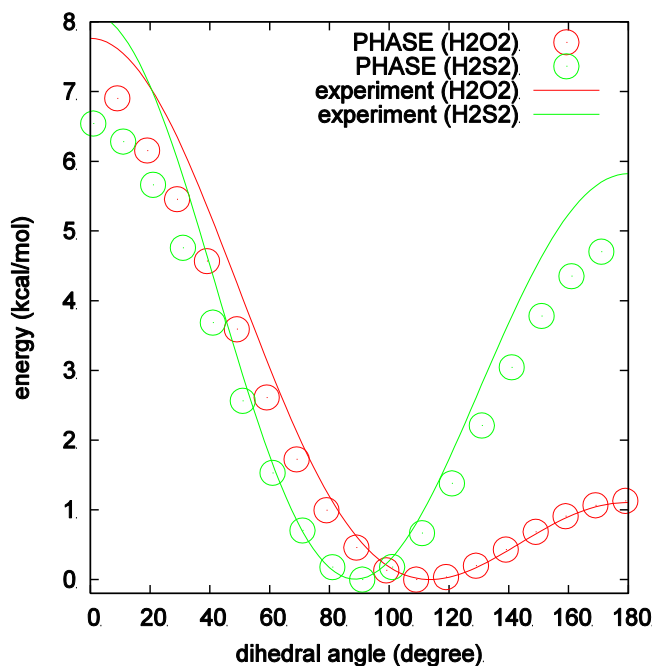
図 5.49 H 2 O 2 およびH 2 S 2 分子の2面角とエネルギーの関係
