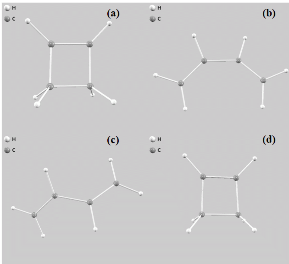
図 5.56 Meta dynamics シミュレーションによって得られた分子構造のスナップショット。(a): バイアスポテンシャル 2 回更新 (b) バイアスポテンシャル 690 回更新 (c) バイアスポテンシャル 1,500 回更新 (d) バイアスポテンシャル 18,070 回更新
