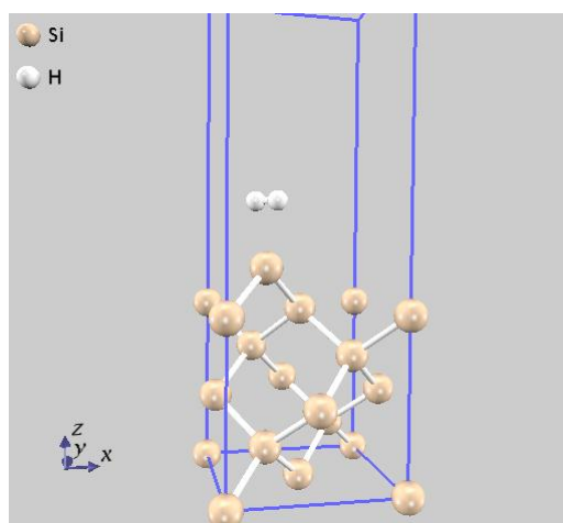
図 5.47 遷移状態における原子配置
