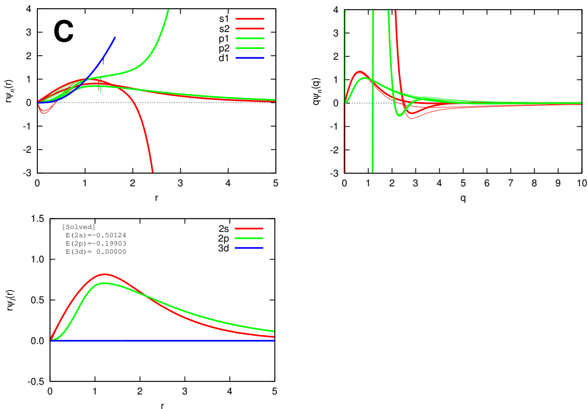
図 5: 炭素原子のウルトラソフト擬ポテンシャル (p.1): 波動関数 (左上), 波動関数の Fourier 変換 (右上), 解き直した波動関数 (左下) を表示しています。左上図では, 波動関数は s は束縛軌道と非束縛軌道の 2 種類, p は束縛軌道と非束縛軌道の 2 種類, d は非束縛軌道となります。矢印はカットオフ半径を示しています。非束縛軌道は途中までしか表示していません。左下図では, 擬ポテンシャルを解き直した結果なので束縛軌道のみが表示されます。解かれた固有エネルギーの値も記入されます。右上図は波動関数の Fourier 変換であり, ゼロとなる q 値が波動関数のカットオフエネルギーの目安になります。
