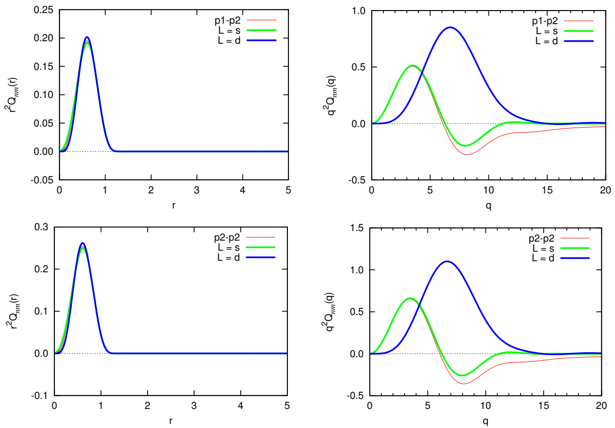
図 15: 炭素原子のウルトラソフト擬ポテンシャル (p.11): デフィシット電荷密度関数 (左) とその Fourier 変換 (右) を表示しています。赤線が全電子デフィシット電荷密度, 緑線が擬デフィシット電荷密度です。緑線の Fourier 変換がゼロとなるところが電荷のカットオフエネルギーの目安となります。
