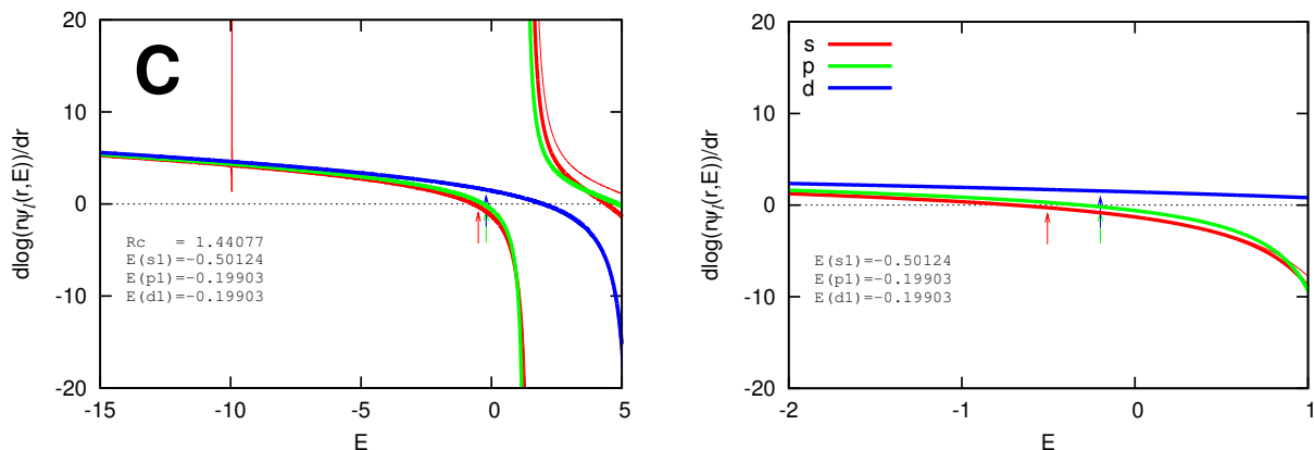
図 2: 炭素原子のノルム保存擬ポテンシャル (p.2): 波動関数の対数微分を表示しています。左図はエネルギーの広い範囲, 右図は固有エネルギー付近の表示となります。矢印は参照エネルギーを示しています。表示された R_c は対数微分をとる半径, エネルギーは参照エネルギーの値です。細線が全電子波動関数, 太線が擬波動関数であり, 両者が一致していることが望ましいです。左図で細線が発散していないところで太線が発散している場合は ghost 状態が存在することが考えられます。
