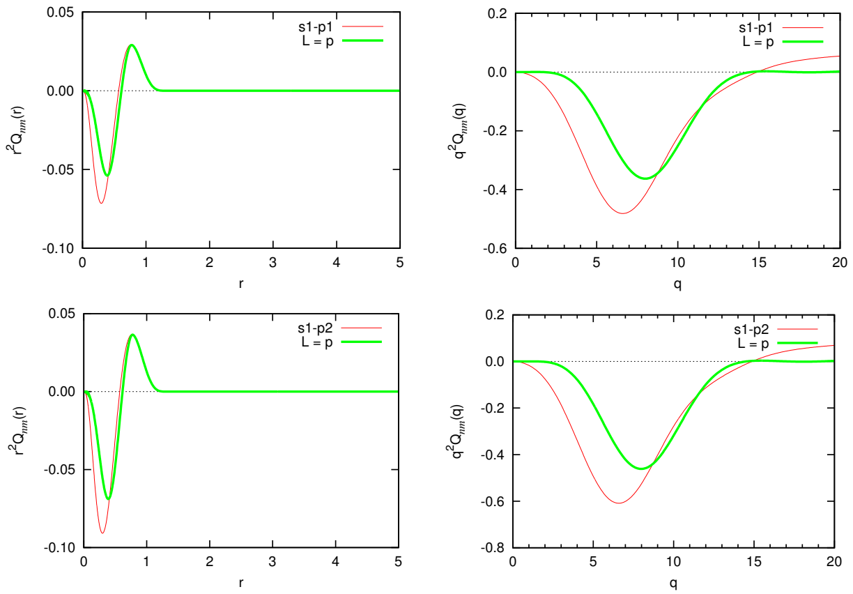
図 12: 炭素原子のウルトラソフト擬ポテンシャル (p.8): デファイント電荷密度関数 (左) とその Fourier 変換 (右) を表示しています。赤線が全電子デファイント電荷密度, 緑線が擬デファイント電荷密度です。緑線の Fourier 変換がゼロとなる場所が電荷のカットオフエネルギーの目安となります。
